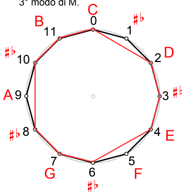
3° modo di M.
