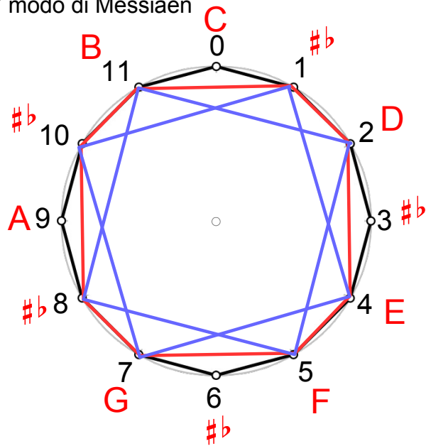
2° modo di Messiaen
